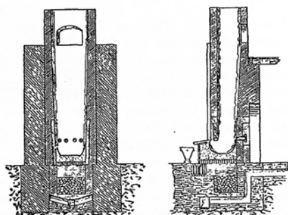
Stolberger Ofen
