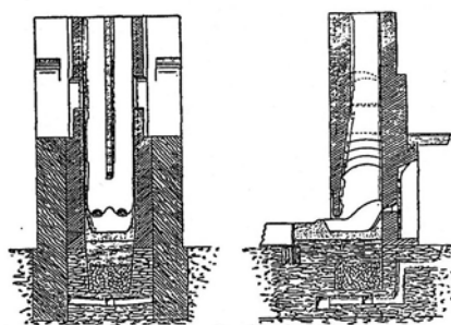
Wellnerscher Doppellofen.
