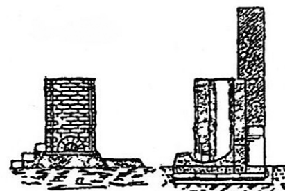
Schönlebscher Krummofen.
