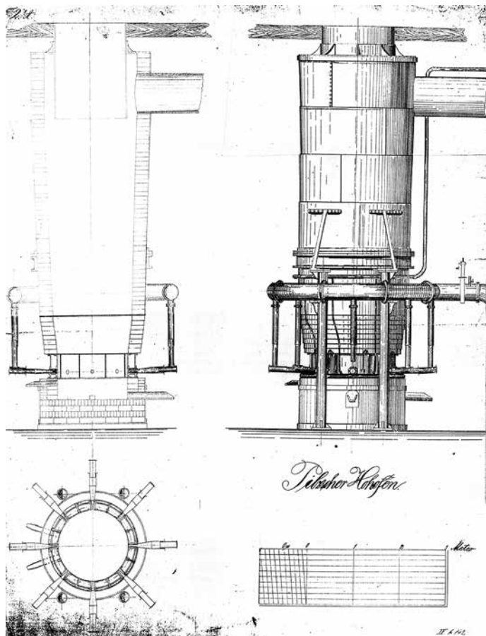
Pilscher Schachtofen Skizze.
