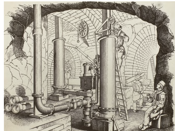
Diese Wassersäulenmaschine in der „Alten Mordgrube“ (Brand-Erbisdorf) hatte Brendel 1823/24 gebaut (Zeichnung von Eduard Heuchler 1857). Sie diente dazu, Wasser aus dem Schacht zu pumpen. Zwei solcher Maschinen von Brendel sind im Segen Gottes Erbstolln (Roßwein) zu besichtigen.
