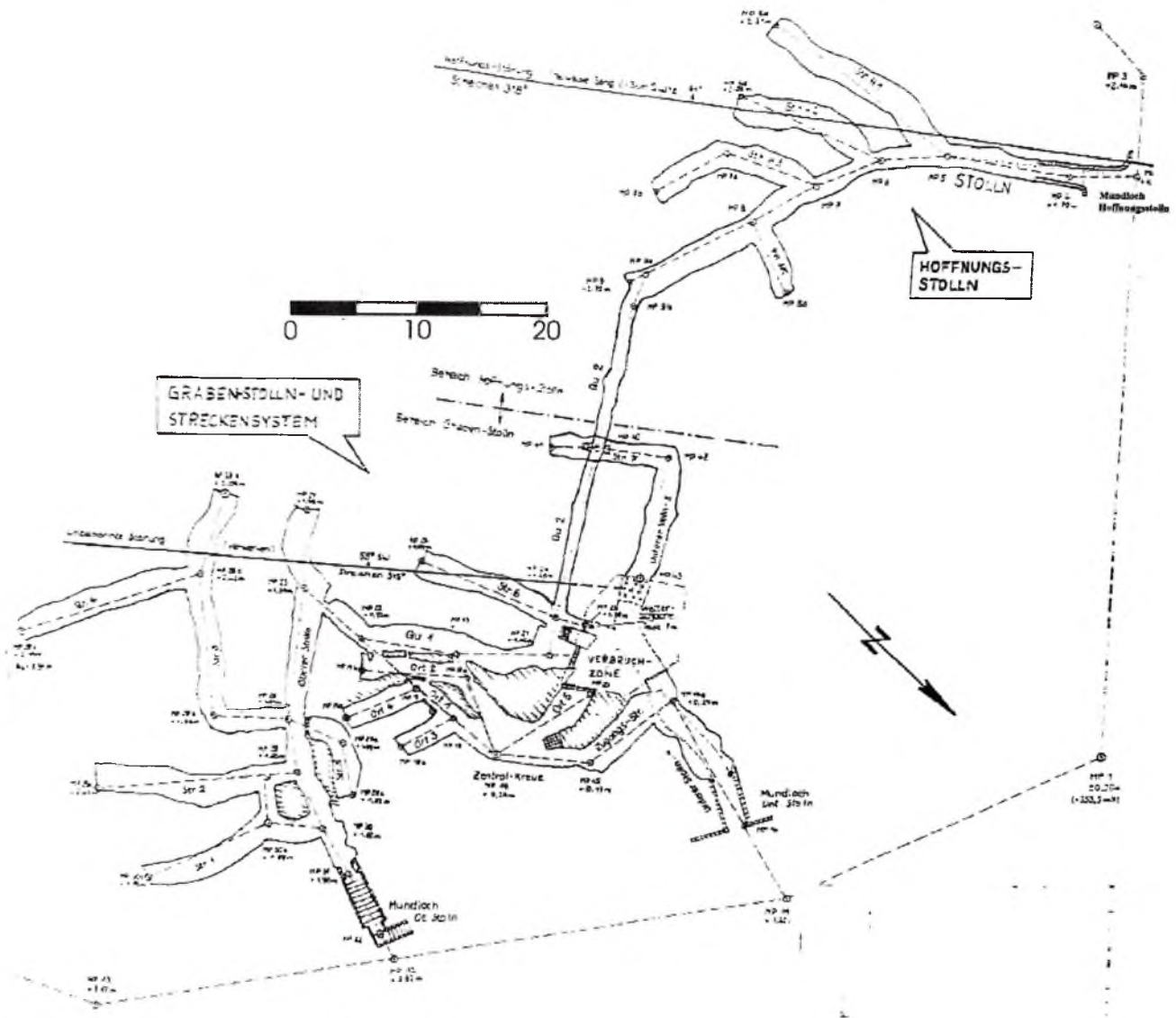
Riss des „Stollnsystem am Graben“ (Abbildungen: Archiv Kirchberger Bergbrüder)
